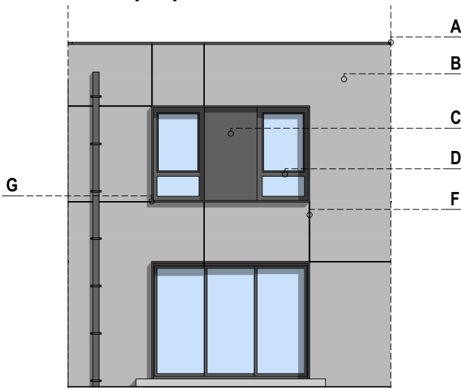
Elewacja Tylna
